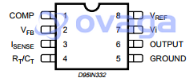
Minidip/SO8
